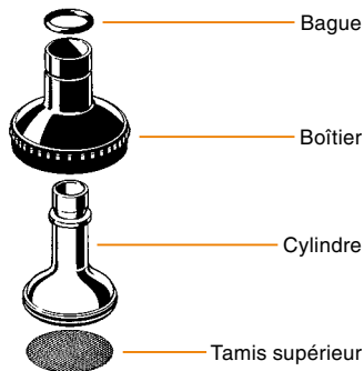
Repousser le Cylindre du Couvrecle pour le sortir du Boîtier
